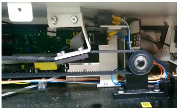
Medidor de COF Labthink (correa suelta, pieza metálica dañada, suciedad)
